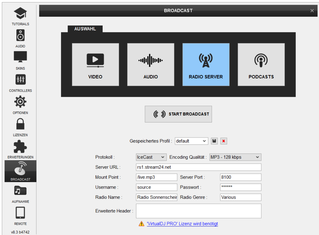
Abb. 5: VirtualDJ | Radio Server Parameter
